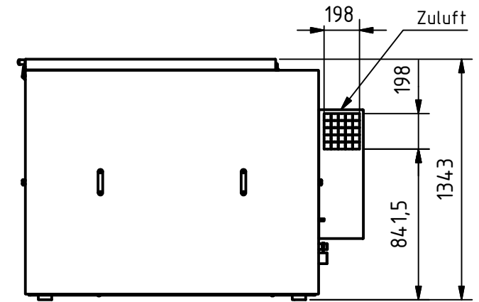
Seitenansicht ( 1 : 25 )
