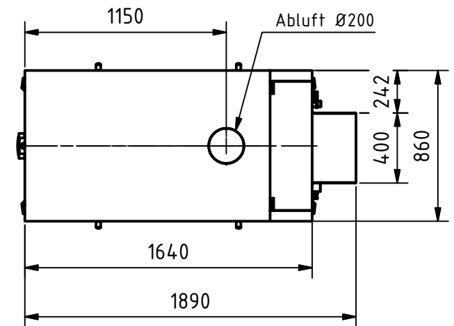
Draufsicht ( 1 : 30 )
