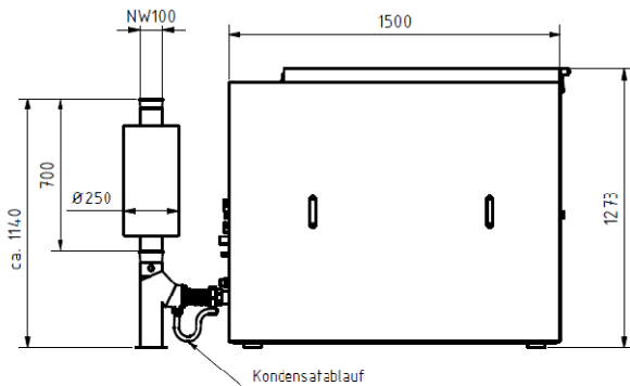
Abb.: Abgasführung – Beispiel KWE 20G-4 AP
