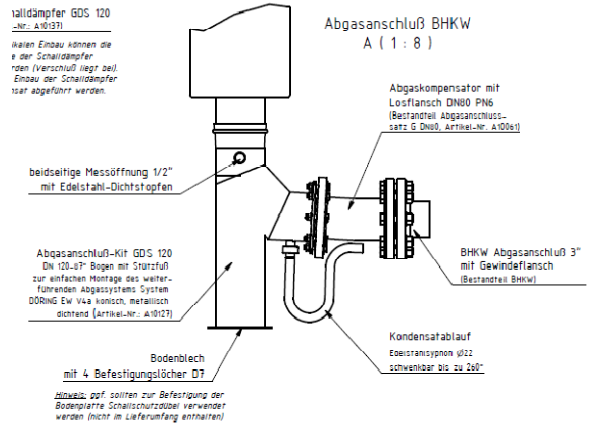
Abb.: Abgasanschlußkit – Beispiel KWE 48G-4 SPN
