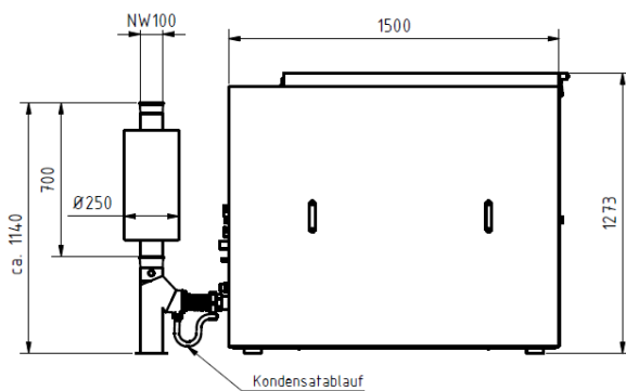
Abb.: Abgasführung – Beispiel KWE 12G-4 AP
