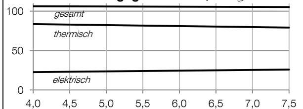
Wirkungsgradkurven [% / kW el ]
