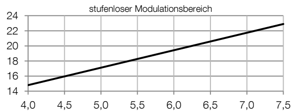
Leistungskurve [kW th / kW el ]
