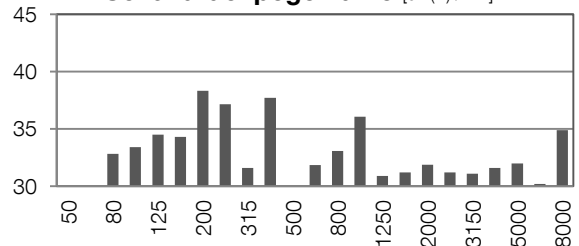
Schalldruckpegelkurve [dB(A) / Hz] 5)
